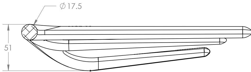
SECTION A-A SCALE 1 : 2
